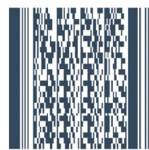
PDF417
