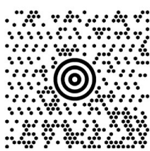
Maxicodes
